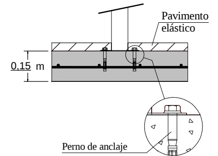
DETALLE CIMENTACIÓN para suelo de caucho
