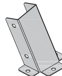
80250 Anclaje chapa
