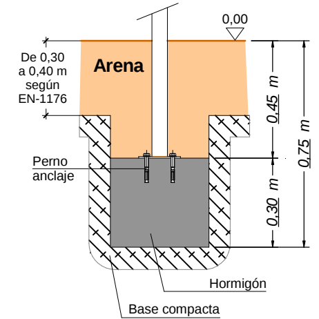
DETALLE CIMENTACIÓN para arenero
