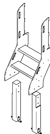
7 Escalera arenero x1 +anclaje arena 58113502 x2
