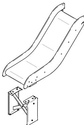
6 Tobogan pequeño x1 +anclaje arena 80615 x1
