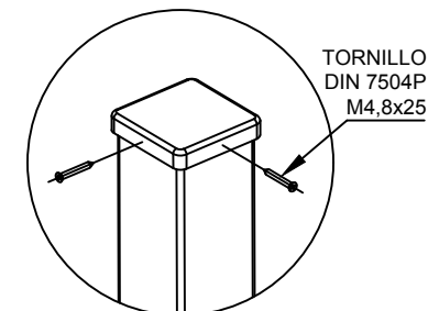
DETALLE Colocación tapa
