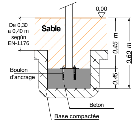
DÉTAIL DE FONDATION pour bac à sable
