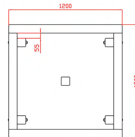
Vista Planta
